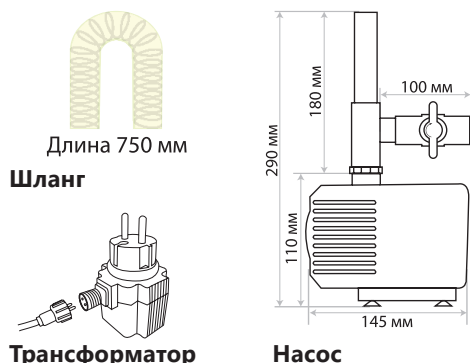
Фонтанная установка в сборе
